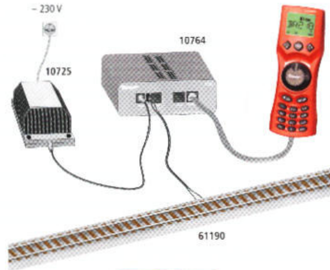
Aufbau des Roco Digital Systems (Europa-Version mit 230 V) mit der multiMAUS
